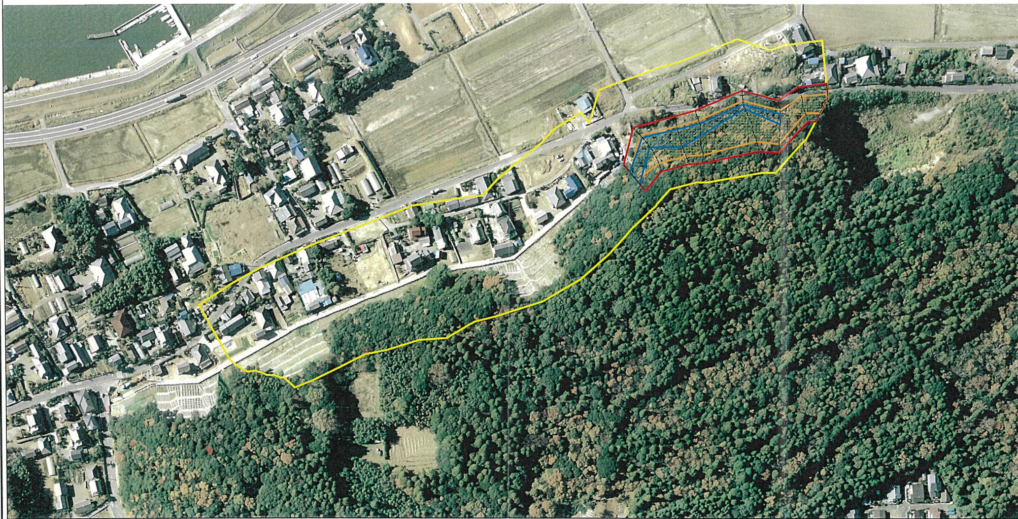
様式-2-1(急) 土砂災害警戒区域・土砂災害特別警戒区域 区域図(その2)
