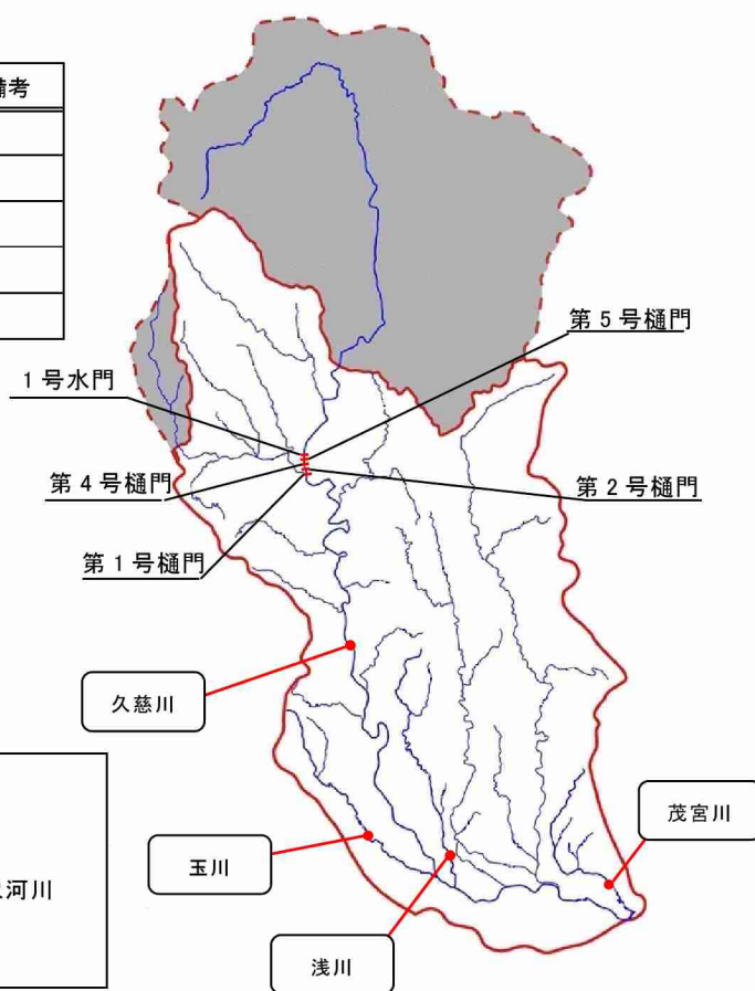
10 11 12 13 14 15 16 17 18 19 20 21 22 23 24 25 図・2.5 主な河川管理施設の位置図
