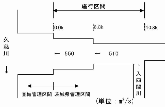
図・2.3 各河川の流量配分図及び代表断面図 (2)
