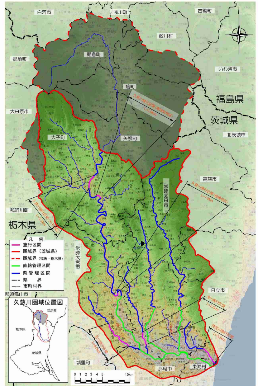
図-2.1 河川工事施行区間
