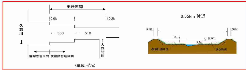
図-2.3 各河川の流量配分図及び代表断面図 (2)
