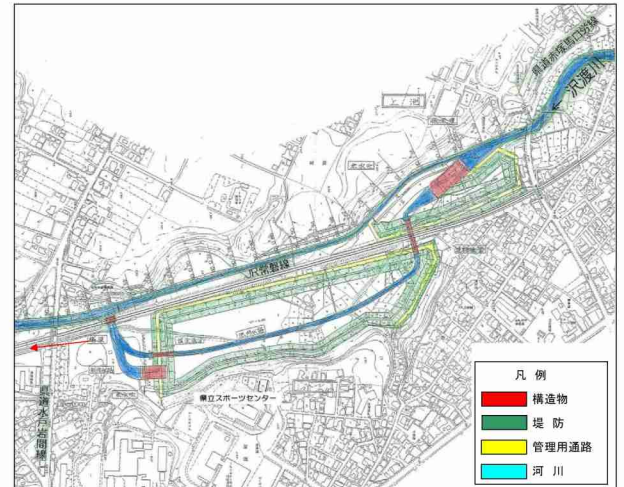
調節池概要図(沢渡川)
