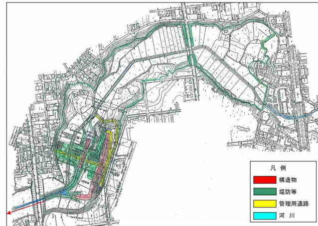
調節池概要図(中丸川)
