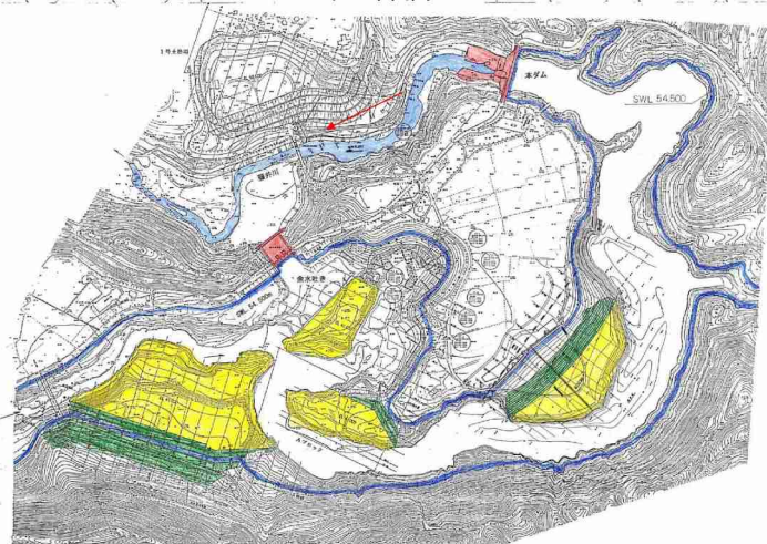
ダム平面図
