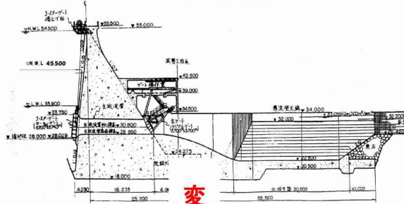
ダム縦断面
