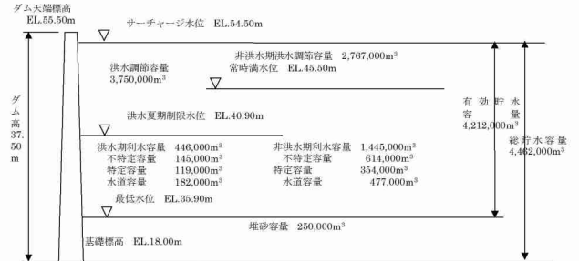
貯水池容量配分図 (再開発)
