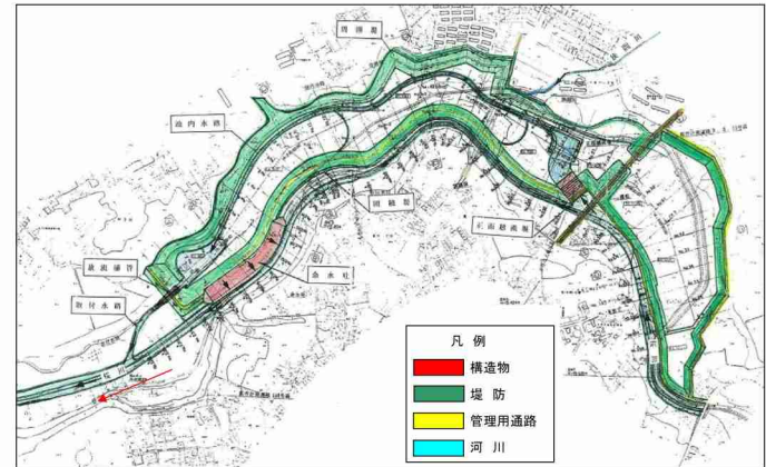
調節池概要図(桜川)
