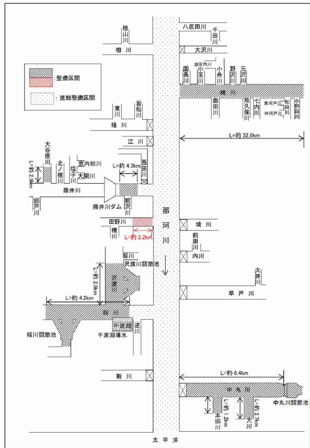
図 2-2 那珂川圏域河川整備状況模式図
