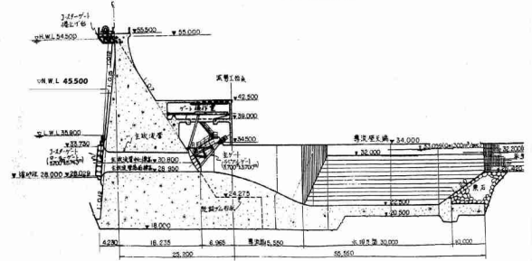
ダム縦断面
