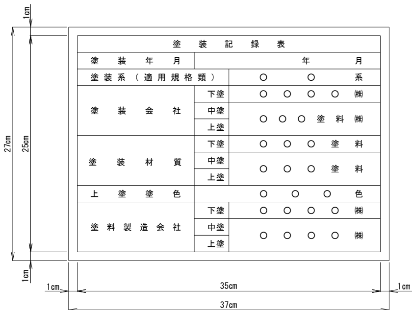
図-3-2-3 塗装記記録表の仕様
