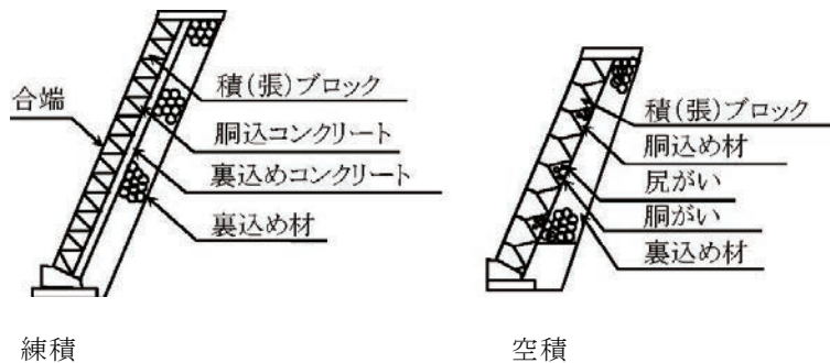
図3-2-5 コンクリートブロック工
