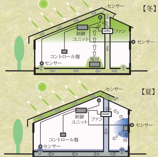
パシブソーラーシステムのイメージ
