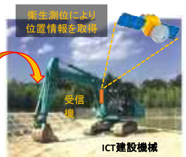
3次元設計データを建設機械に搭載
