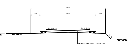
支線道路 (碎石舗装) 11号 S=1:30
