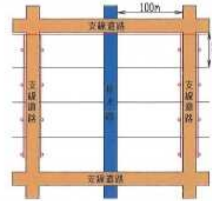
支線排水路 S=1:30
