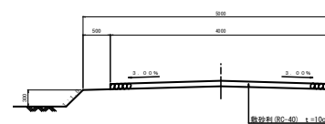
支線道路 (碎石舗装) 1号~10号 S=1:30
