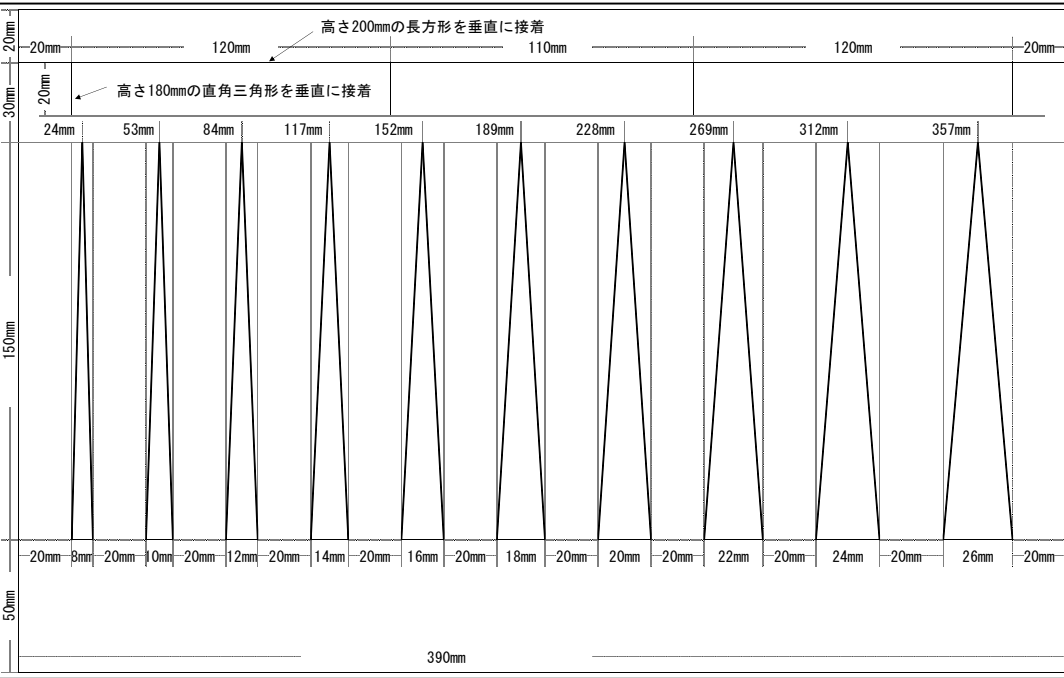
スリット製図
