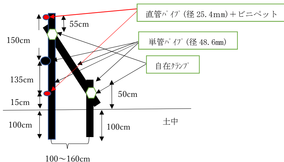
図2 側面図
