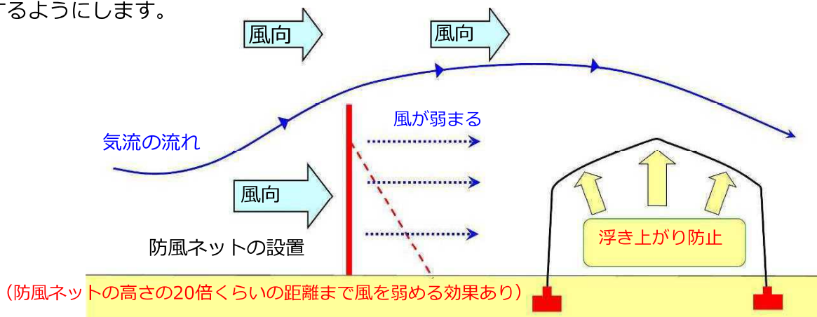
図-20 防風施設（防風ネット）の設置
