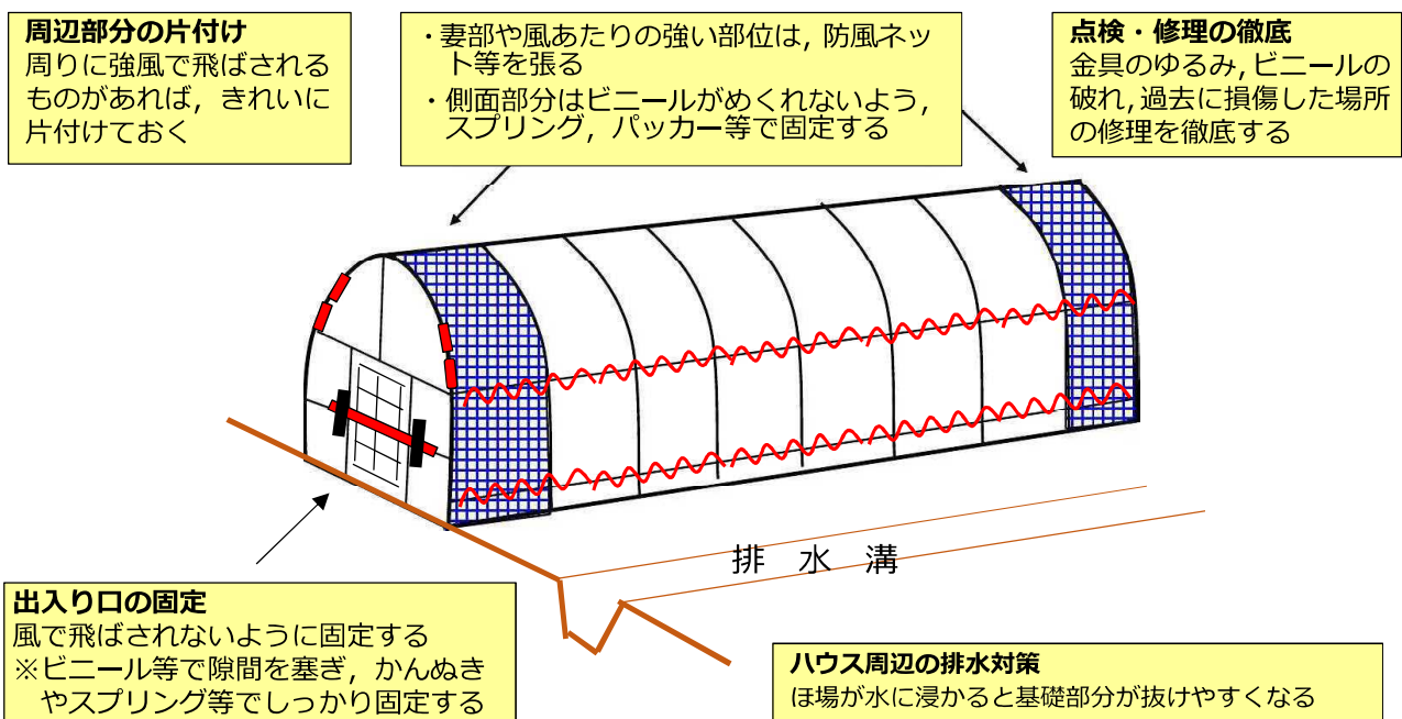
図-23 パイプハウスの強化事例
