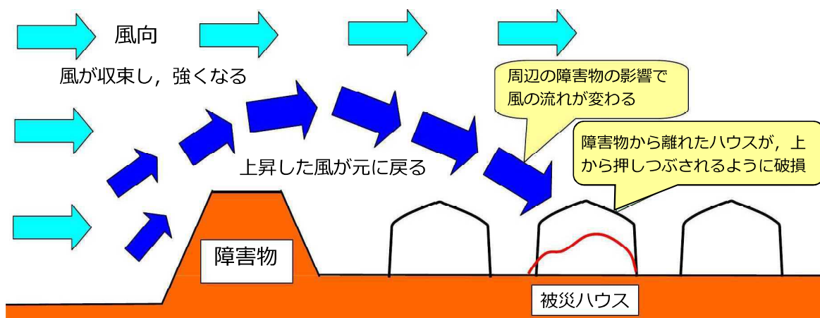
図-8 周辺の地形や障害物により風の流線が変化する事例
