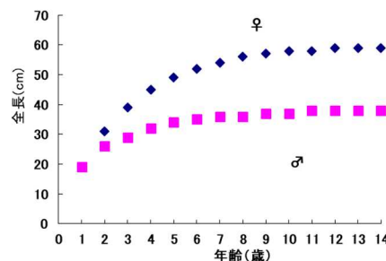
図 1 イシガレイの成長
