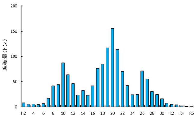
図 2 イシガレイの漁獲量(属地、水試システム)
