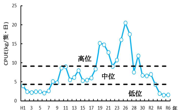
図 3 イシガレイの CPUE(固定式刺網(建網))
