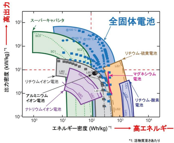
図 4 各種蓄電デバイスのエネルギーと出力の関係を示すラゴンプロット。既存のリチウムイオン電池やスーパーキャパシターと、現在開発が進められている各種革新電池（ナトリウムイオン電池、アルミニウムイオン電池、マグネシウムイオン電池、リチウム空気電池）の特性に加え、本開発の全固体セラミックス電池の特性を併せて示す。既存のリチウムイオン電池やキャパシターが達成できていない高出力と高エネルギーを兼ね備えた領域（右上の領域）を、開発した全固体電池が可能にしている。出力特性とエネルギー密度とを兼ね備えた蓄電デバイスが初めて開発できた。特にリチウムイオン電池との比較では、出力特性がほぼ3倍以上である。また、現在開発が進んでいる各種革新電池（ナトリウムイオン電池やリチウム空気電池、マグネシウム電池、アルミニウム電池など）と比較しても、全固体電池がエネルギーと出力特性を兼ね備えた優れた電池系であることを示している。
