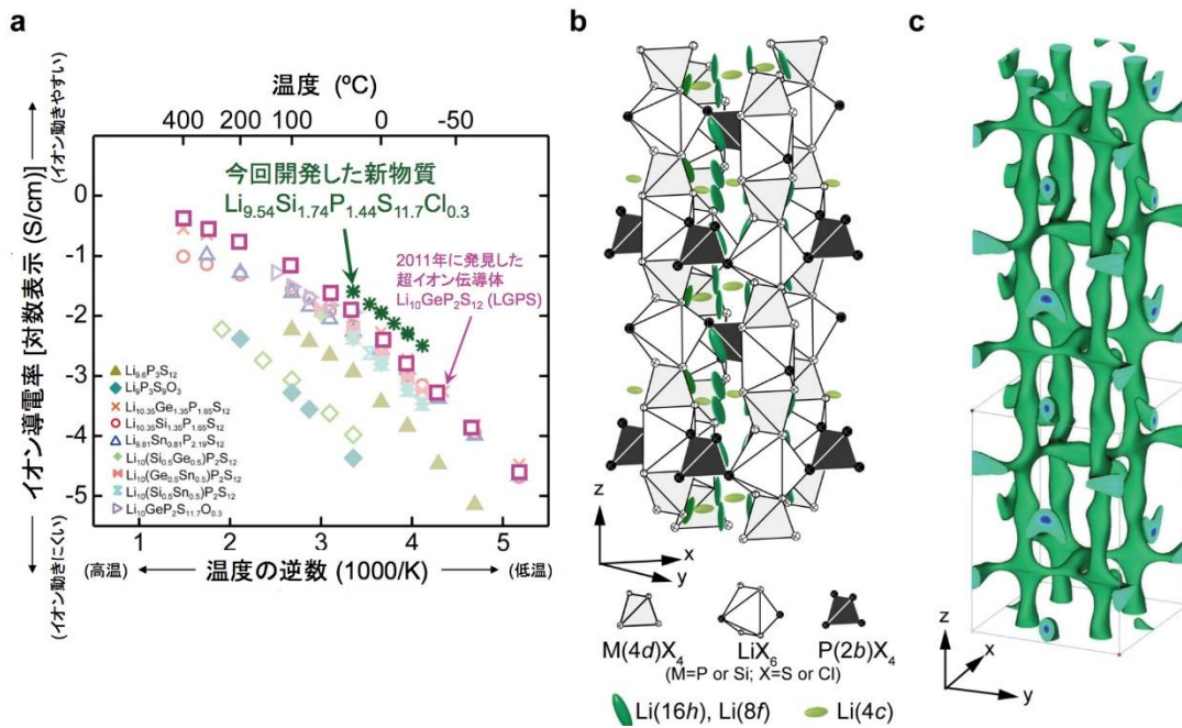
図1 a 今回発見した超イオン伝導体 ( \text{Li}_{9.54}\text{Si}_{1.74}\text{P}_{1.44}\text{S}_{11.7}\text{Cl}_{0.3} と \text{Li}_{9.6}\text{P}_3\text{S}_{12} ) のイオン伝導率の温度依存性を従来のリチウムイオン伝導体 \text{Li}_{10}\text{GeP}_2\text{S}_{12} とその類似構造を持つ物質と比較して示す。発見した \text{Li}_{9.54}\text{Si}_{1.74}\text{P}_{1.44}\text{S}_{11.7}\text{Cl}_{0.3} のリチウムイオン伝導率は室温 (27 °C) で 25 \text{ mS cm}^{-1} を示し、従来のリチウムイオン伝導体 \text{Li}_{10}\text{GeP}_2\text{S}_{12} ( 12 \text{ mS cm}^{-1} ) の2倍の伝導率を示す。 b, c 今回発見した超イオン伝導体 \text{Li}_{9.54}\text{Si}_{1.74}\text{P}_{1.44}\text{S}_{11.7}\text{Cl}_{0.3} の結晶構造とイオン伝導経路。この構造は大強度陽子加速器施設 J-PARC に設置された茨城県材料構造解析装置 (iMATERIA) を用いて明らかにした。b は全体の構造、c は一次元のリチウムイオン伝導経路を示す。b ではリチウムイオンの熱振動の様子を示す。リチウムイオンは上下方向に非常に大きく熱振動しており、リチウムが超イオン伝導に関与していることがわかる。また、c 図はリチウムが三次元的に連なり、室温での三次元的なイオン拡散を示している。
