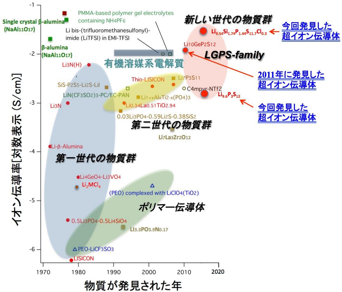
図2 超イオン伝導体の研究の歴史。それぞれの物質が発見された年代とイオン伝導率との関係を示す。第一世代の材料は、イオンが固体中を高速で動き回ることを追求する過程で探索された。第二世代の材料は実用材料として応用することも加味して開発された物質群。本発見の超イオン伝導体は、LGPS（リチウム・ゲルマニウム・リン・硫黄）グループの中でもイオン伝導率の値が 25 \text{ mScm}^{-1} と最も高く、既存の \text{Li}_{10}\text{GeP}_2\text{S}_{12} より2倍以上のイオン伝導率である。リチウムイオン電池に用いられている有機溶媒系より、はるかに高いイオン伝導率であることもわかる。
