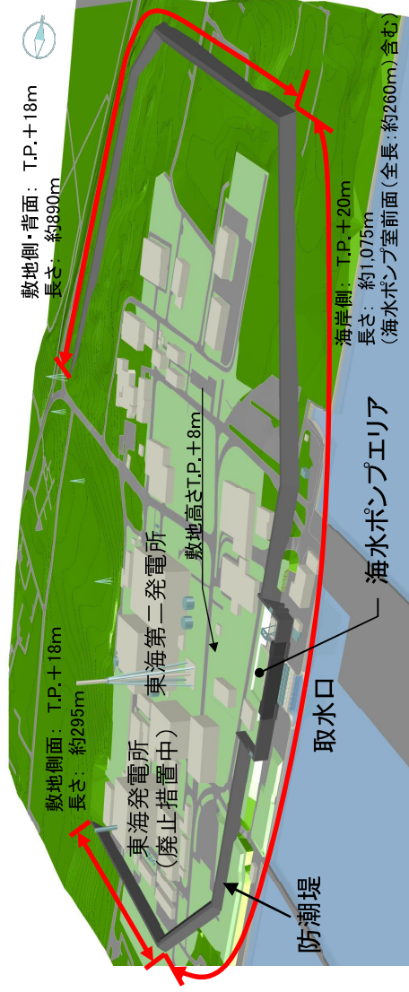
＜防潮堤の概要(イメージ図)＞
