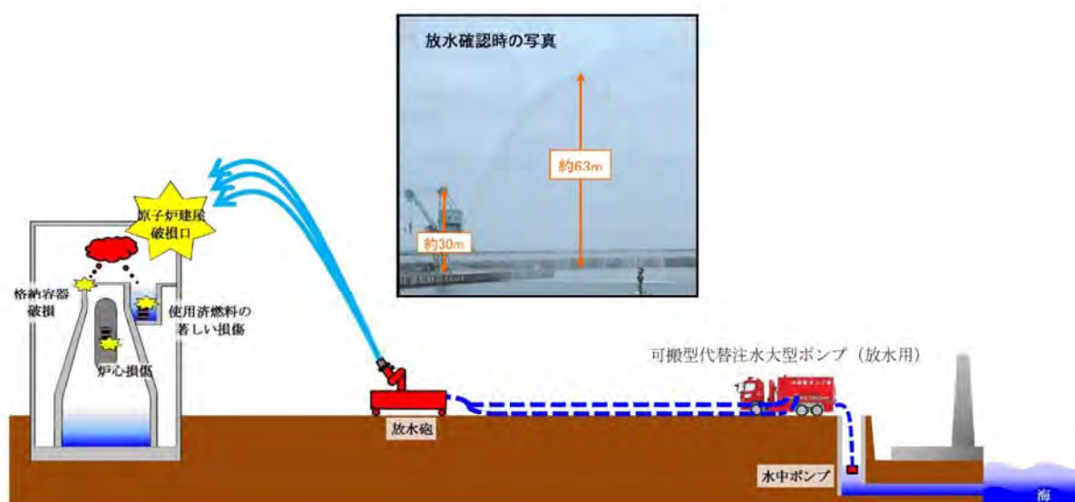
図18.1 放射性物質の拡散抑制対策の概要
