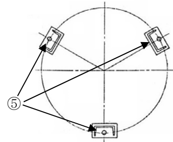
取付ボルト詳細図
