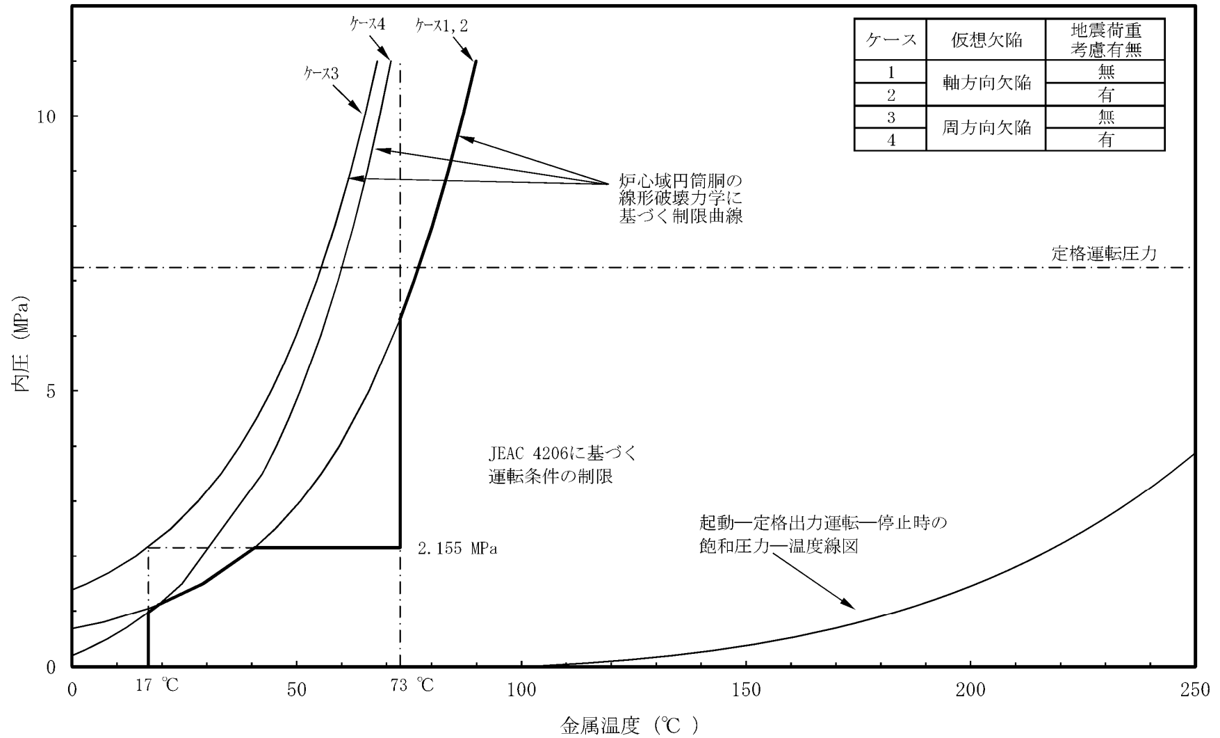
図 3.4-1 原子炉圧力容器の圧力・温度制限曲線（60年時）（炉心領域円筒胴，炉心臨界時）
