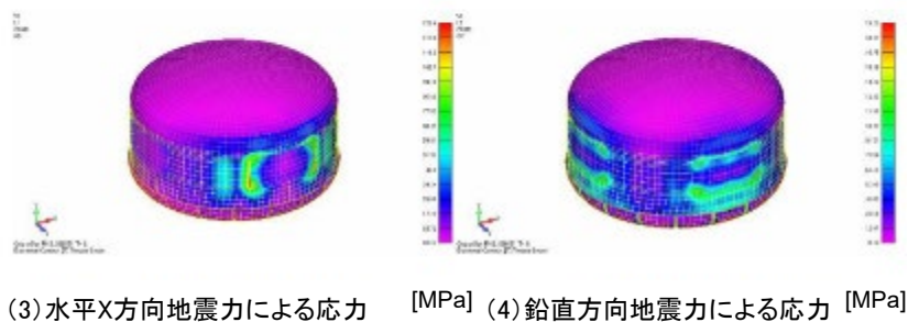
図1 三次元有限要素法による高放射性廃液貯槽の耐震評価例
