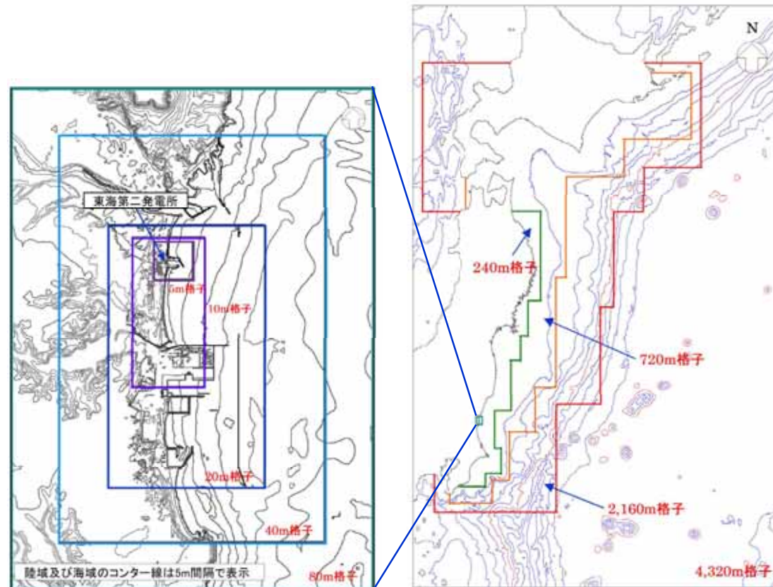
計算領域と格子分割(沖合~沿岸域)
