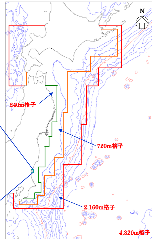
計算格子(沖合～沿岸域)
