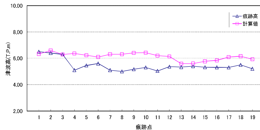
計算値と痕跡高の比較
