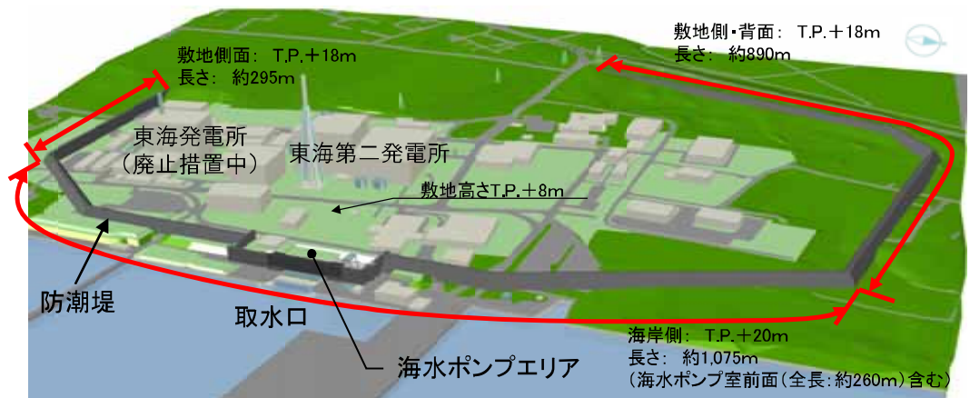
<防潮堤の概要(イメージ図)>
