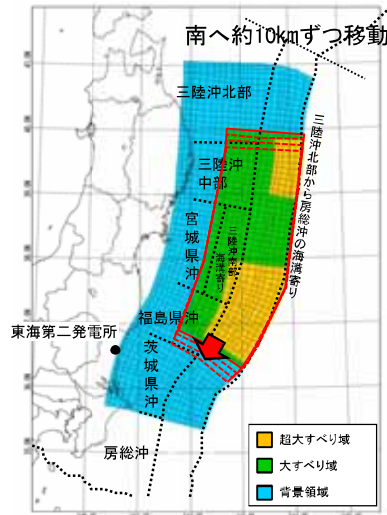
【M9クラスの特性化波源モデル】
