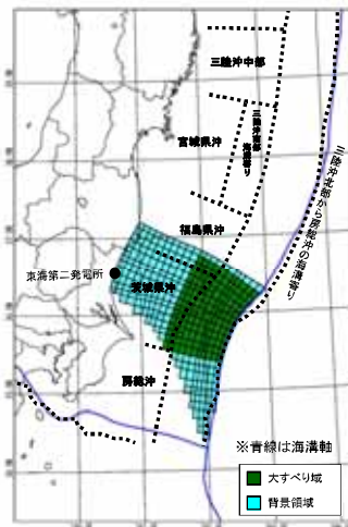
茨城県沖に想定する津波波源
