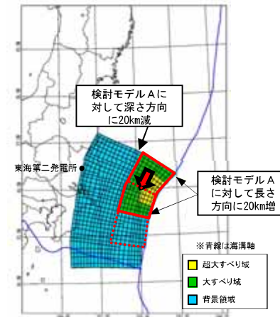
検討モデルB
