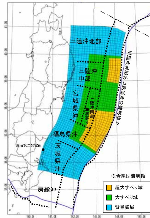
特性化波源モデル(一例)
