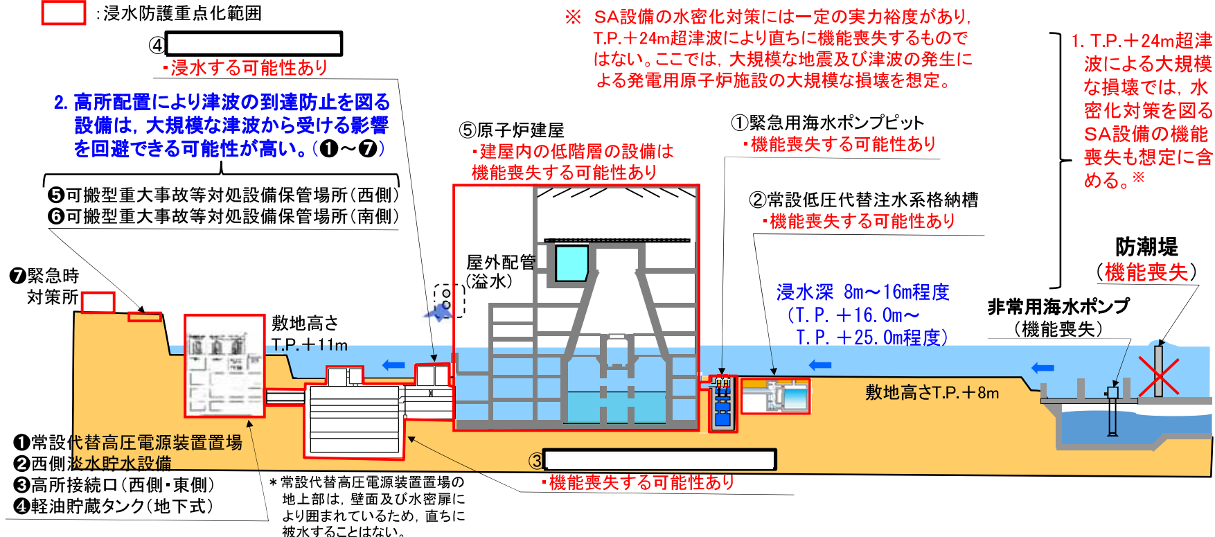
津波区分3のT.P.+24m超津波による発電用原子炉施設の大規模な損壊に対する対応例 津波対策-246
