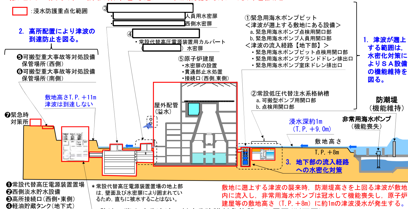
敷地に遡上する津波に対する防護対象施設の配置図(断面図)
