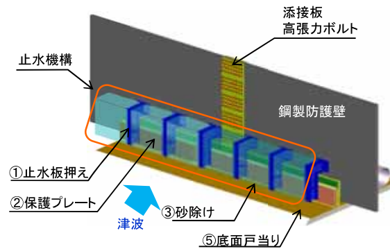
海側から見た止水機構の構造
