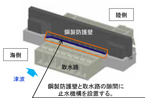
止水機構の設置状況
