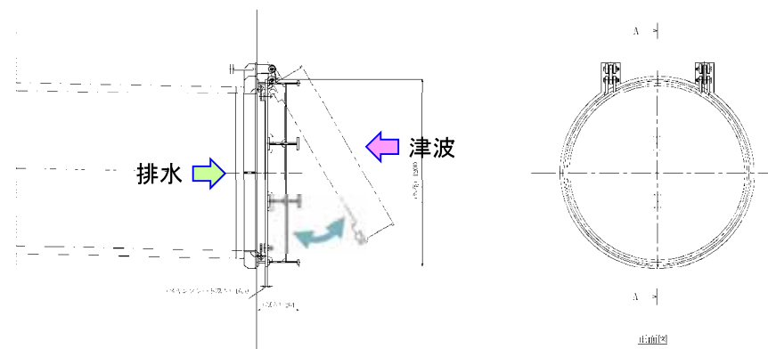
構内排水路逆流防止設備の構造*
