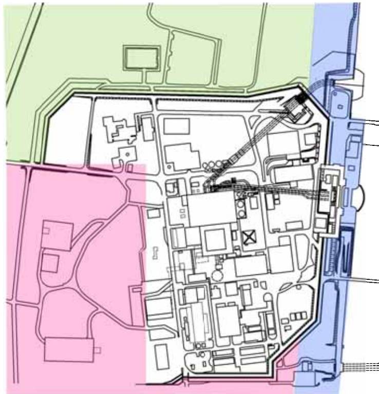
解析において考慮する沈下量
