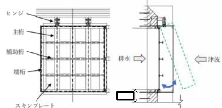
フラップゲートの構造*
