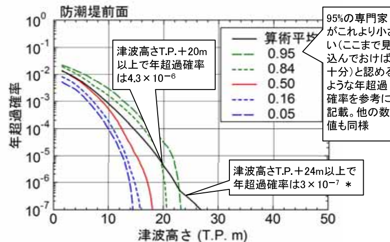
評価に用いる平均津波ハザード曲線
