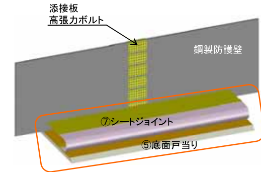
陸側から見た止水機構の構造
