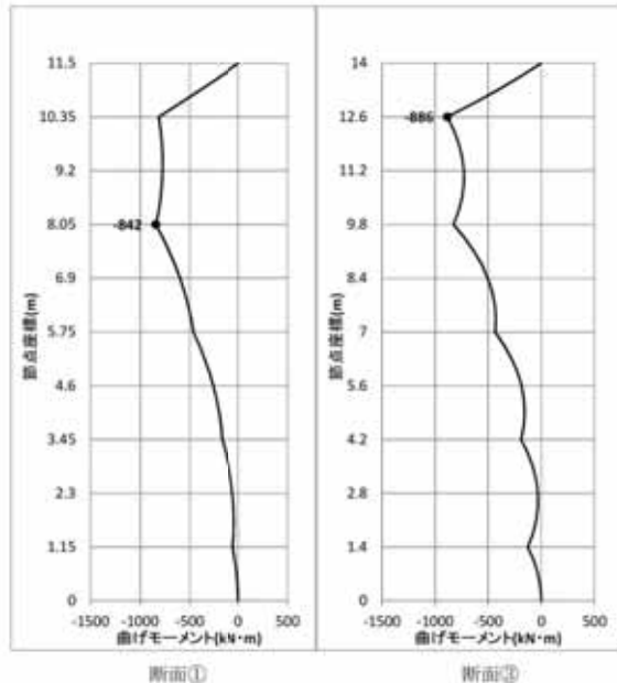
注記：節点距離は鉄筋コンクリート壁の横幅方向の位置を示す。 論点No.32-9参照
