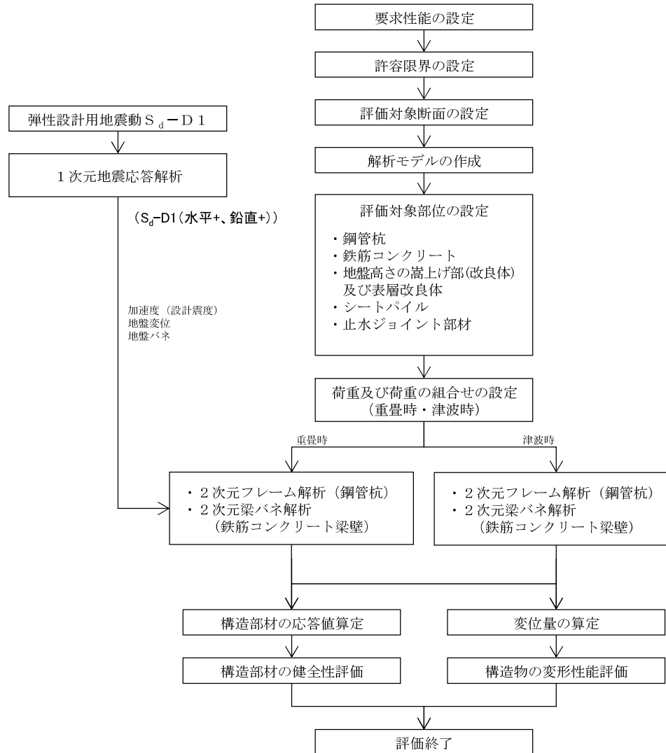
鋼管杭鉄筋コンクリート防潮壁の詳細設計フロー 津波対策-212
