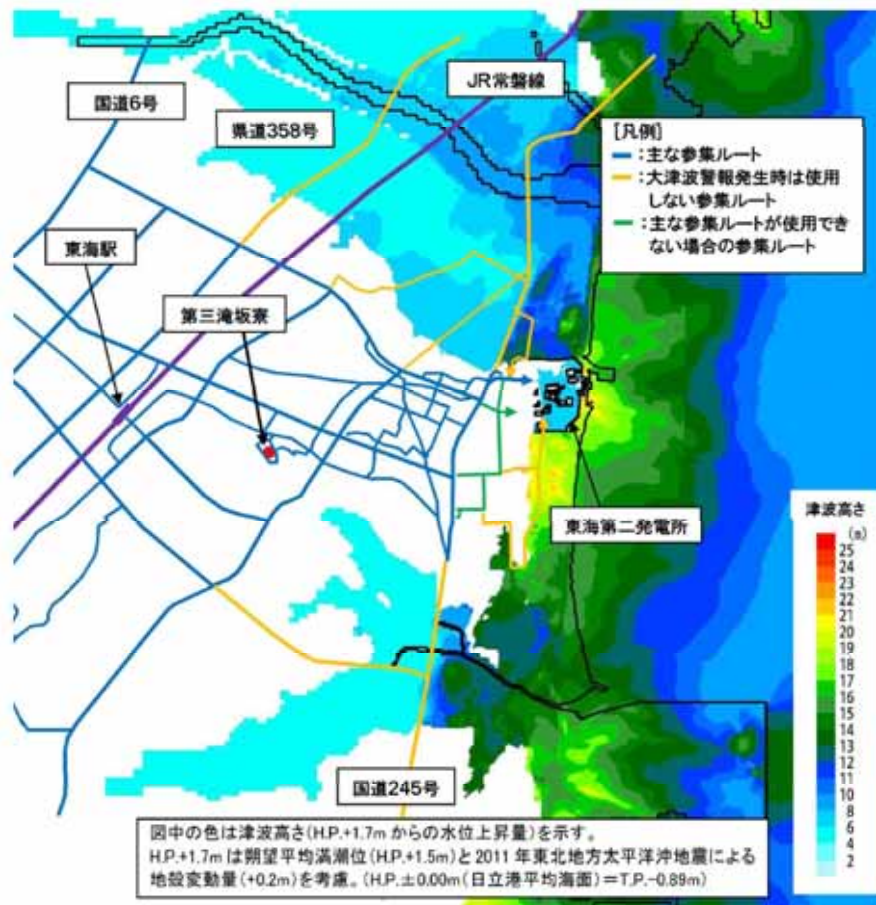
発電所周辺の遡上想定範囲 津波対策-253
