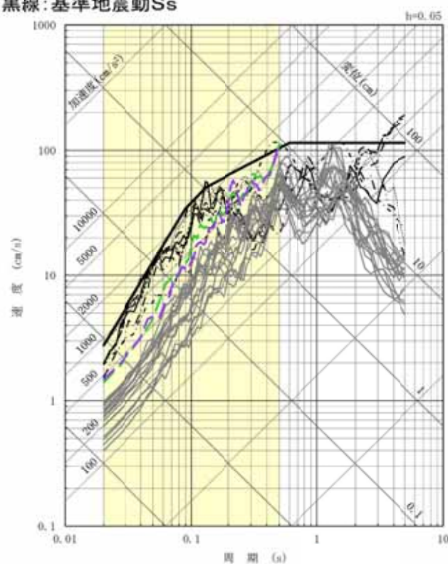
EW方向
