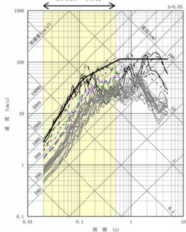
NS方向
