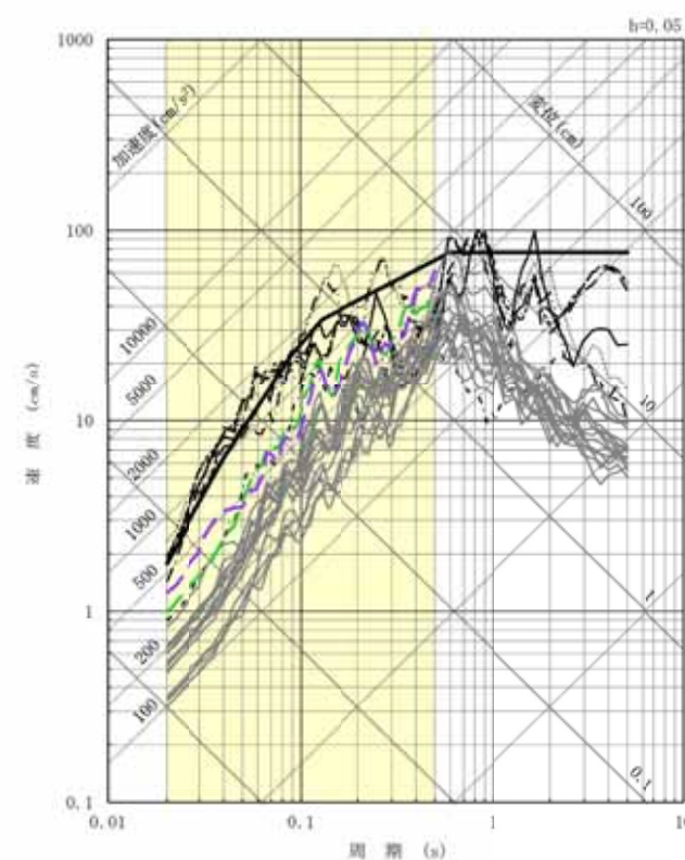
UD方向
