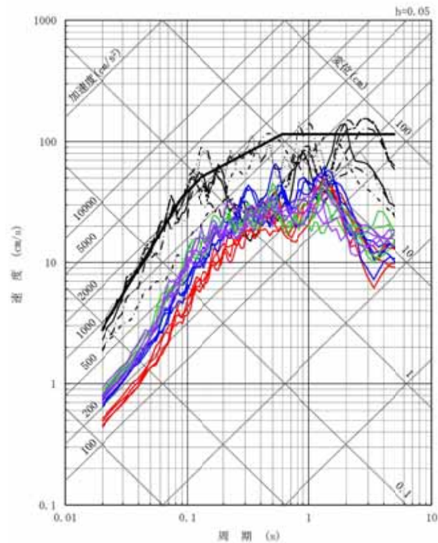
NS方向
