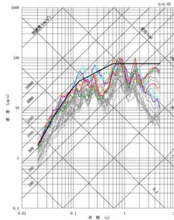
UD成分
