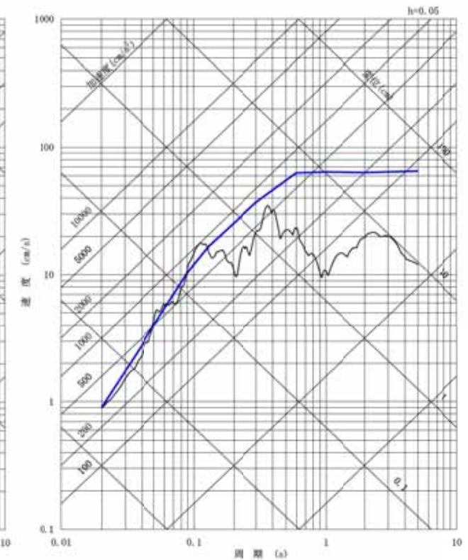
鉛直成分
