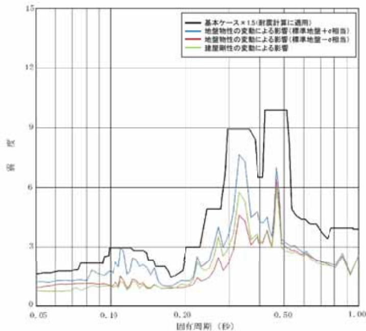
床応答スペクトル (水平方向 h=1.0%)
