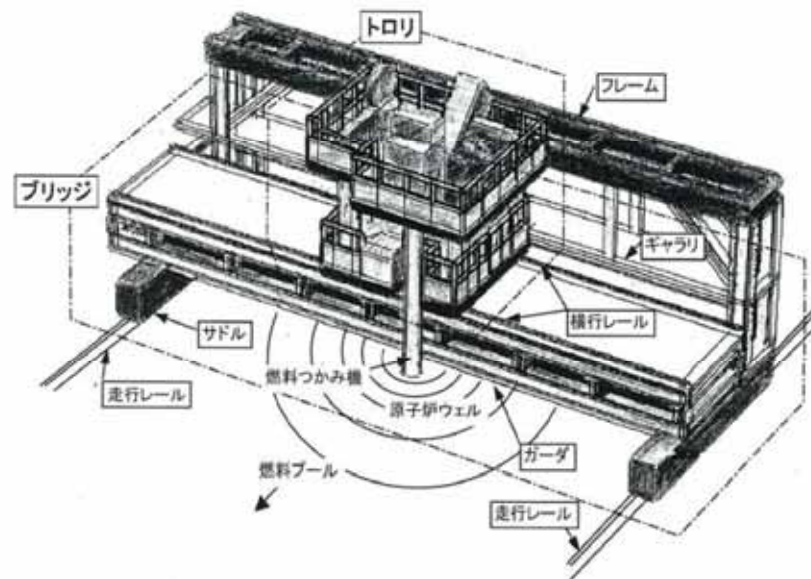
燃料取替機の耐震補強概要図
