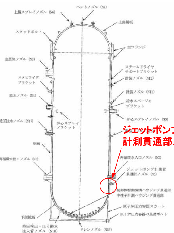
原子炉圧力容器構造概要図
