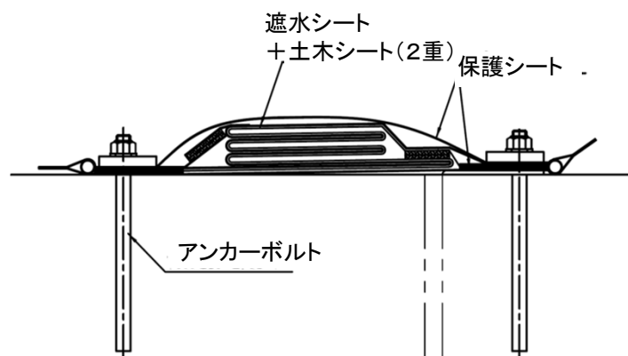
シートジョイント設置図
