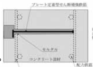
PHb工法の概要
