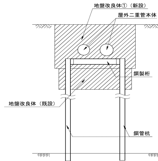
B-B 断面 (杭基礎構造部)
