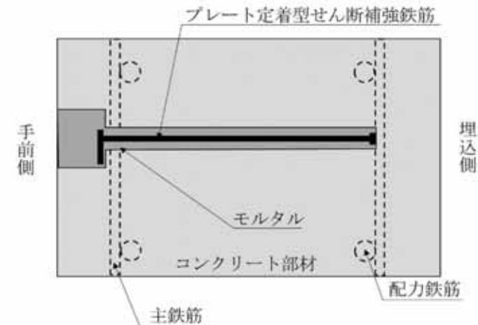
PHb工法の概要
