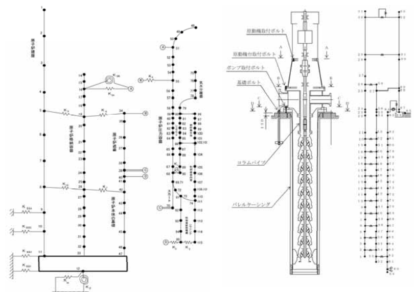
図1 建屋-機器連成解析モデル
