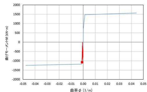
(側壁：貯水機能)
