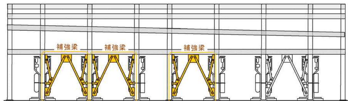
補強構造
