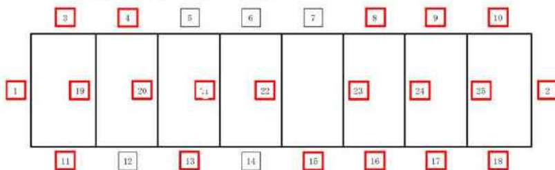
後施工せん断補強筋の適用部材
