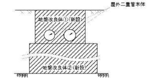
C'-C' 断面 (地盤改良体基礎構造部)
