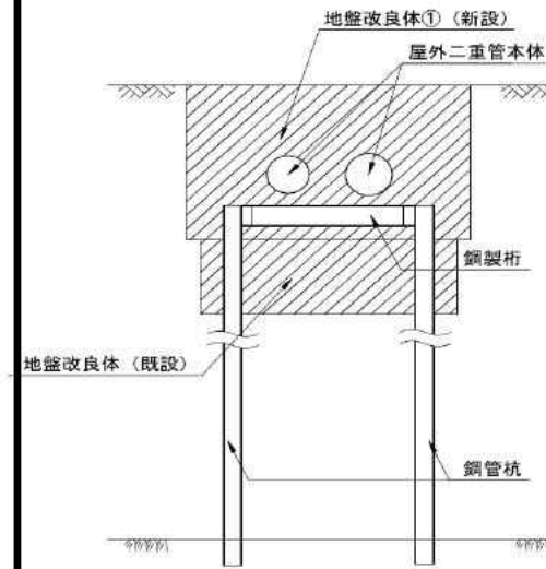
B-B断面 (杭基礎構造部)
