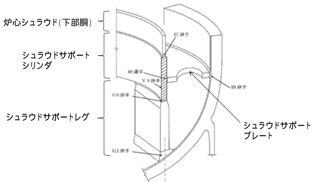
シュラウドサポート概略図
