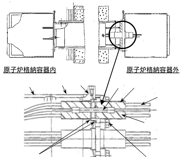
低圧用電気ペネトレーション構造図
