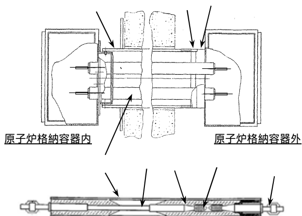
高圧用電気ペネトレーション構造図
