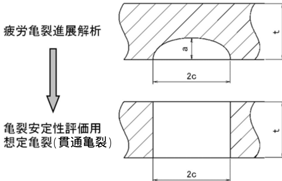
亀裂安定性評価用想定亀裂
