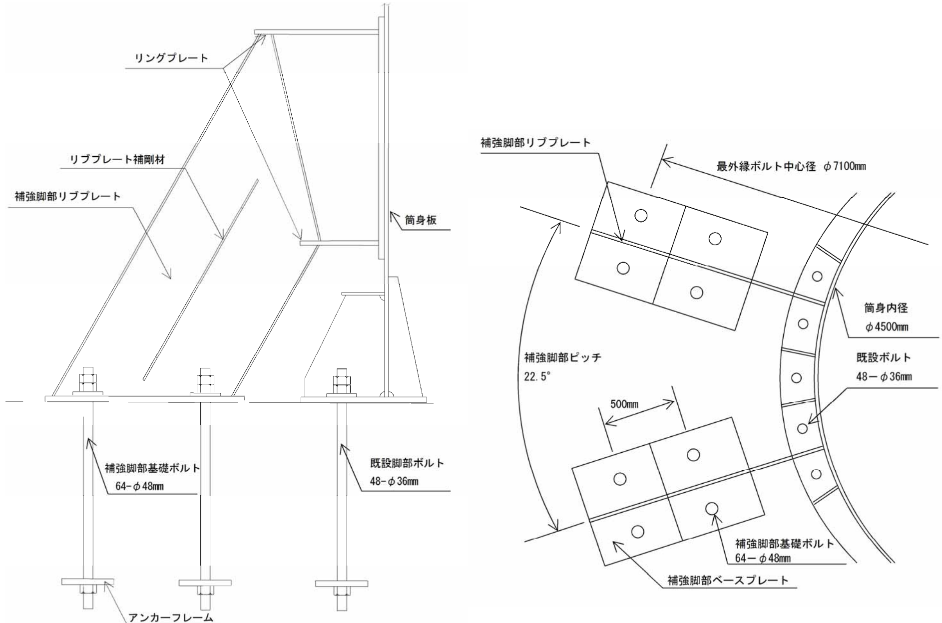
筒身補強脚部概略図
