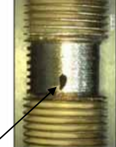
写真③ 主油冷却器(B)伝熱管(1本)漏えい孔
