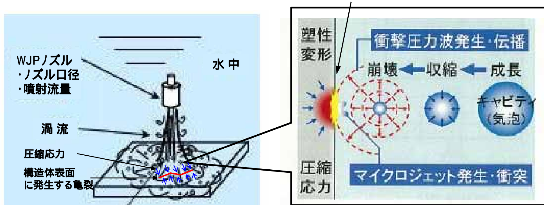
ウォータージェットピーニング(WJP) 施工模式図及び原理
