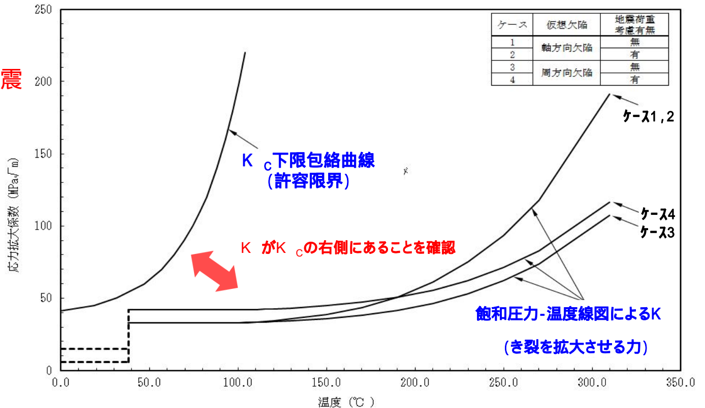
K_{IC} 下限包絡曲線と K 曲線(原子炉压力容器胴:炉心臨界時)
