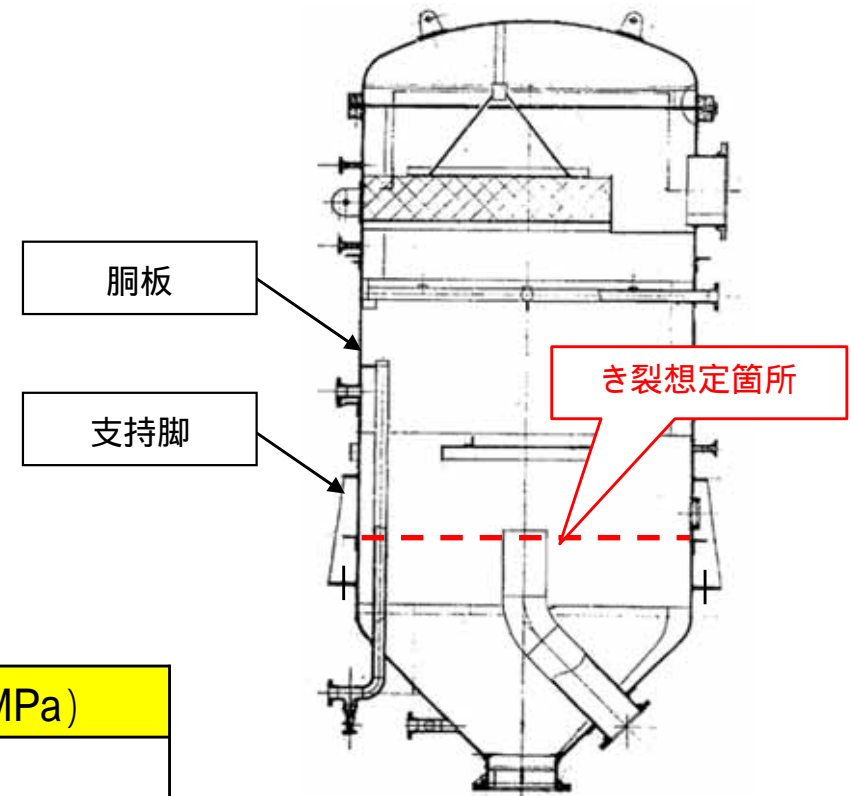
廃液濃縮器蒸発缶構造図
