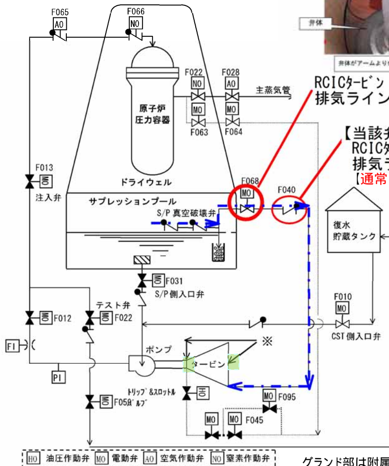
原子炉隔離時冷却系概要図
