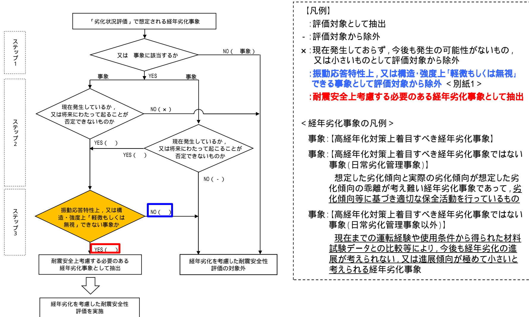
図1 耐震安全上考慮する必要のある経年劣化事象の抽出フロー 高経年化-335
