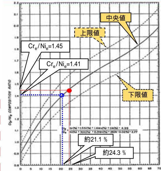
図1 フェライト量導出図 : 原子炉再循環ポンプケーシング : 原子炉再循環ポンプ入口弁
