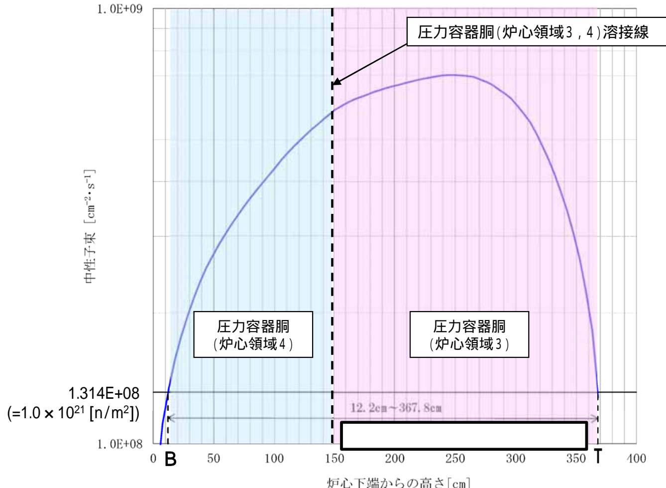
原子炉压力容器内表面における中性子束(E > 1 MeV)の上下方向分布 (運転開始後60年時点で1.0 × 10 21 n/m 2 を超える範囲)
