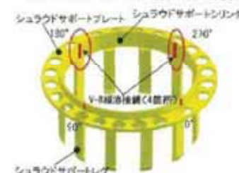
【シュラウドサポート構造図】
