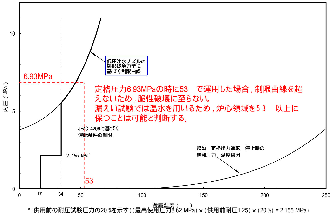
原子炉压力容器の圧力・温度制限曲線(60年時点)(低圧注水ノズル, 漏えい試験時)
