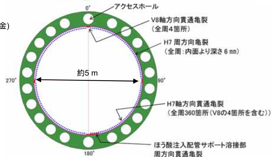
図-2 解析モデル及び亀裂の想定箇所
