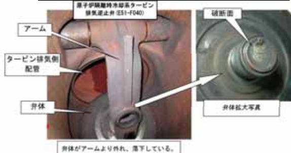
RCICタービン排気ライン隔離弁
