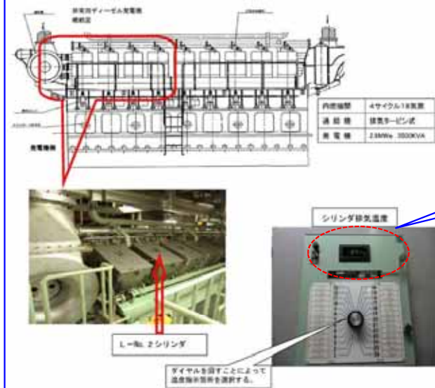
図1 DGシリンダ排気温度のふらつき
