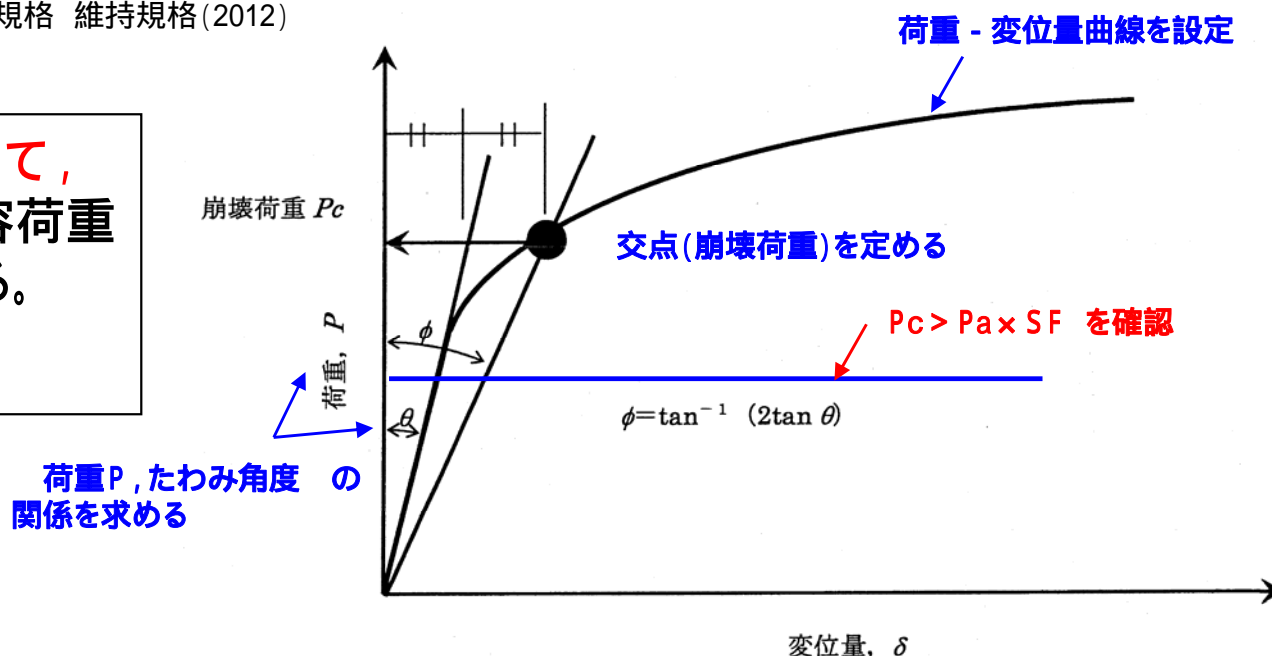
2倍勾配法による崩壊荷重の求め方
