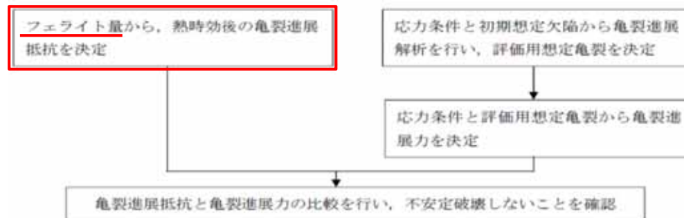
図4 熱時効評価の流れ
