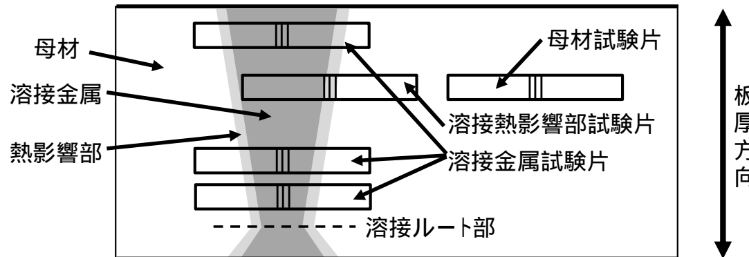
試験片採取イメージ図
