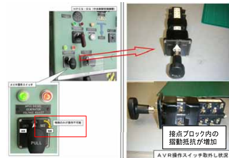
図2 AVR操作スイッチ「増(RAIZE)」方向操作不可
