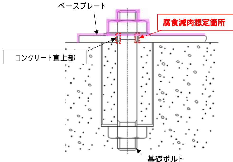
< 基礎ボルト概要図 >
