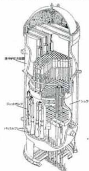
【原子炉压力容器 内部構造図】
