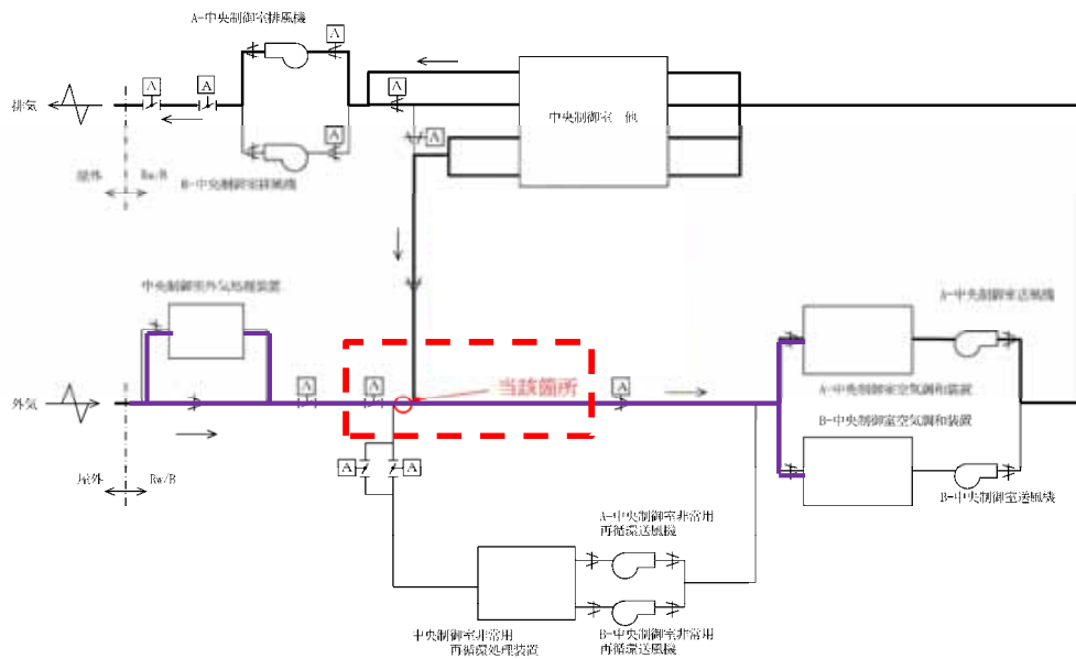
他プラント 中央制御室換気系ダクト腐食部位(概要)
