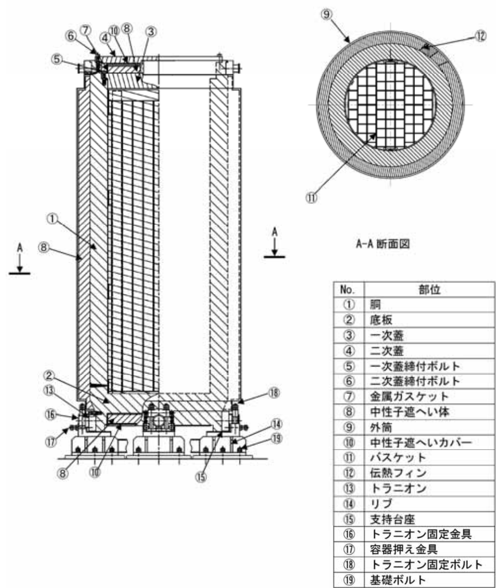
使用済燃料乾式貯蔵容器構造図 (18~21号機)
