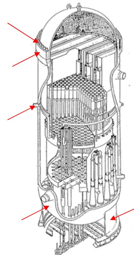
原子炉圧力容器の評価対象
