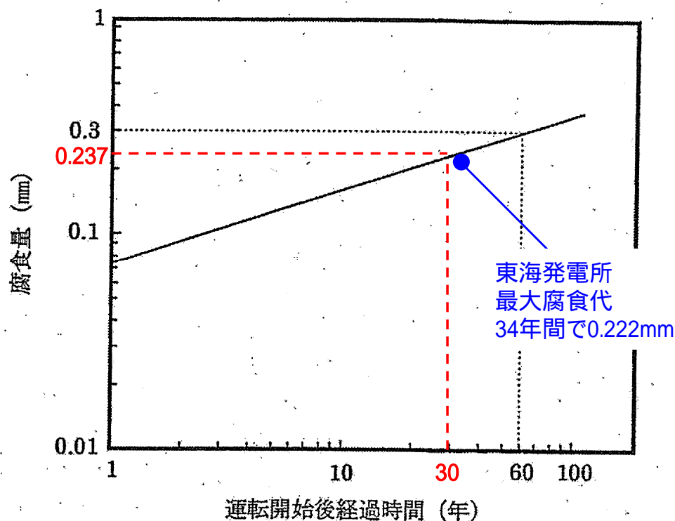
炭素鋼の大気腐食による腐食量
