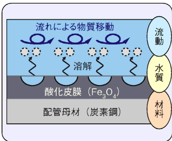
FACによる減肉メカニズム
