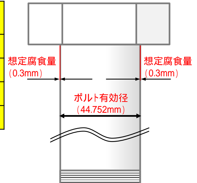
排気筒基礎ボルト(M48)イメージ
