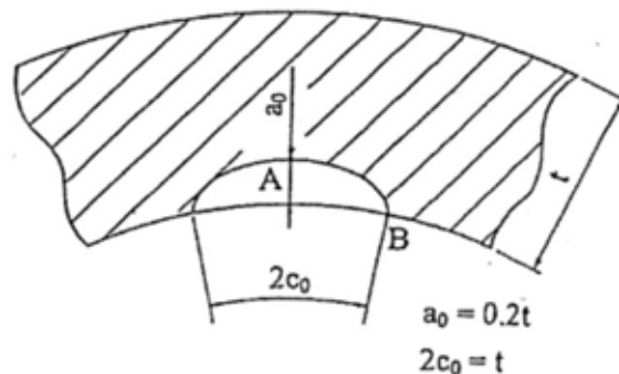
初期欠陥の形状
