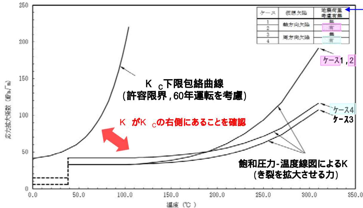
K c 下限包絡曲線とK 曲線(原子炉压力容器胴: 炉心臨界時)
