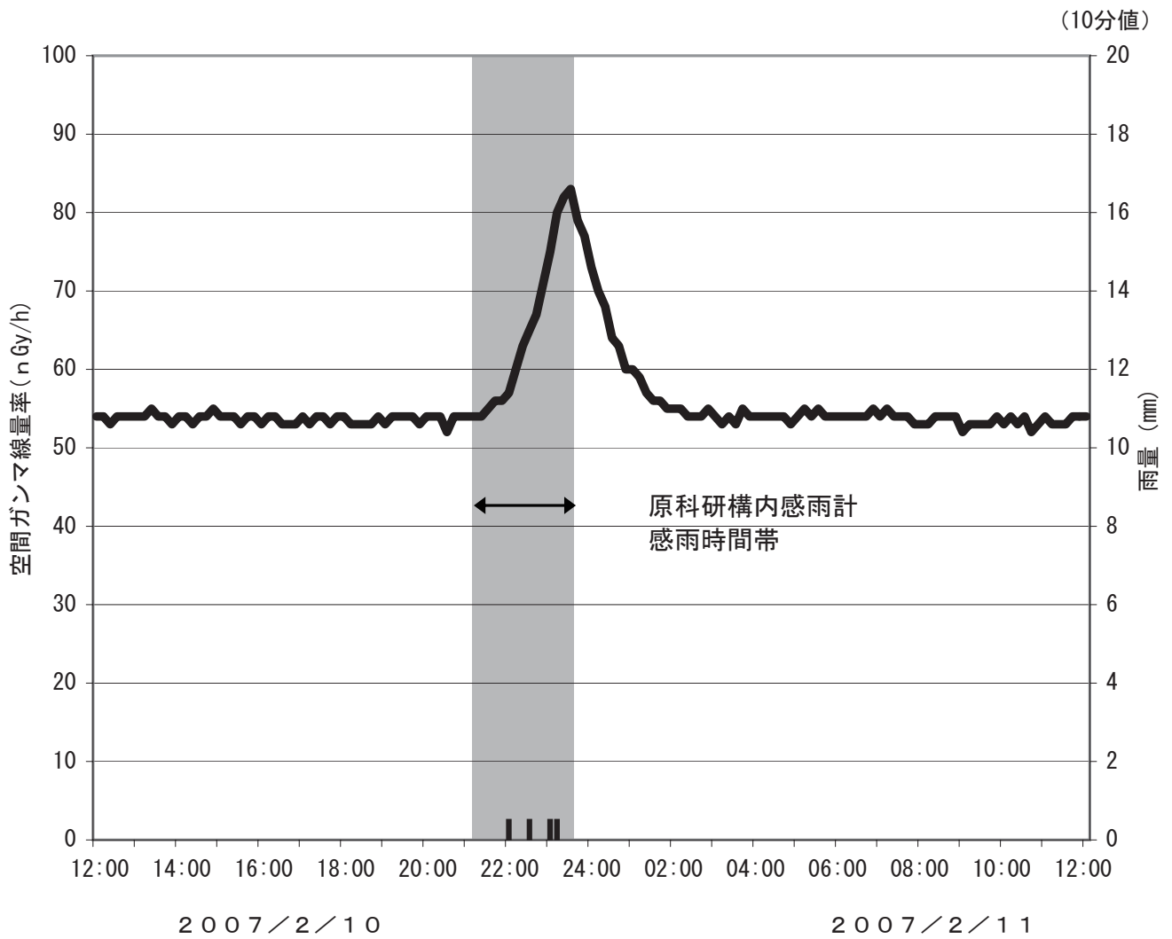
今期の測定の中で最大値が観測された局における空間ガンマ線量率時系列 (東海村亀下)
