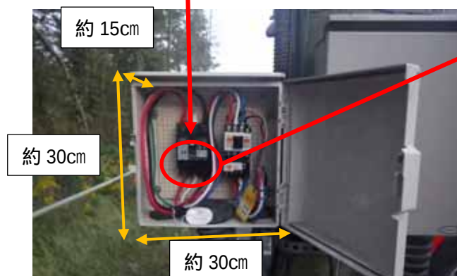
当該照明用電源盤寸法 約 30cm (幅) × 約 30 cm (高さ) × 約 15 cm (奥行)
