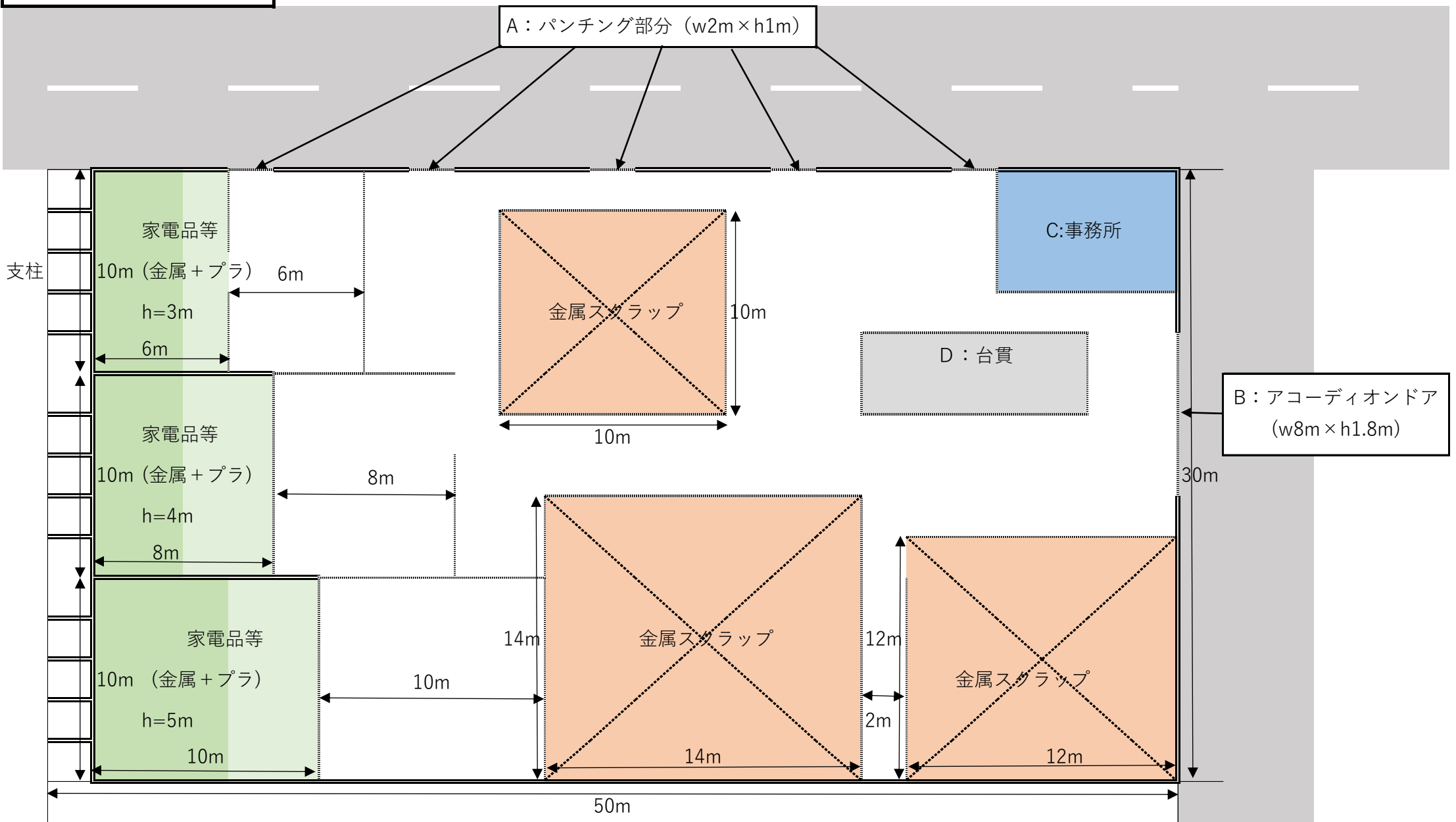
屋外保管事業場平面模式図
