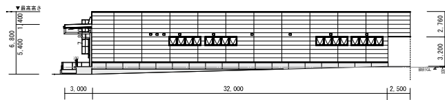
A棟立面図
