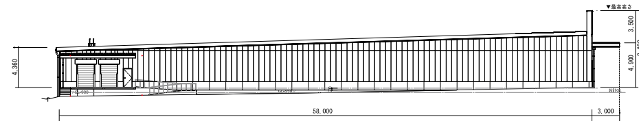
B棟立面図
